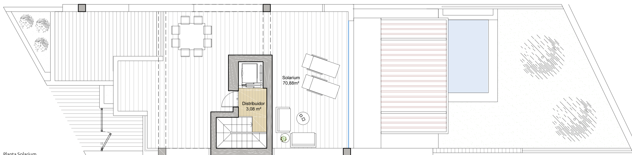
Planta Solarium
